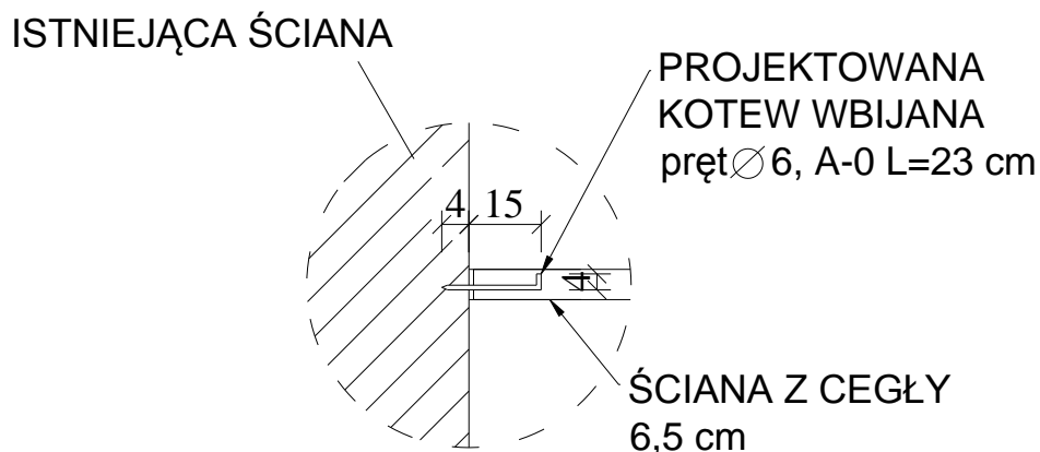
Rysunek 4. Szczegół połączenia ściany działowej z istniejącą ścianą w warstwach 1 i 5
